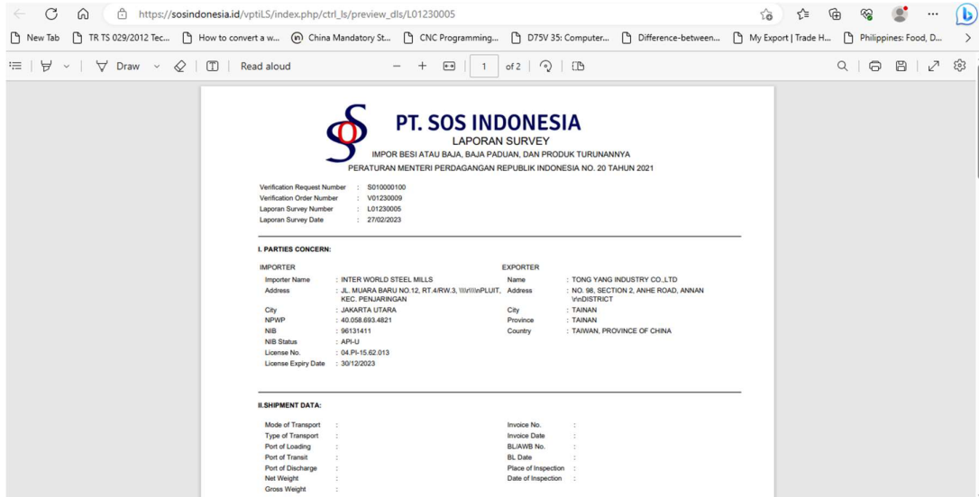
Gambar 30. Preview DLS
